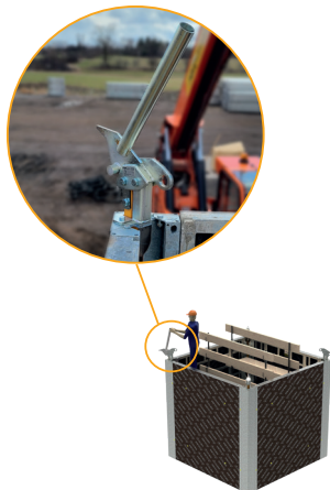
Manuell operasjon
