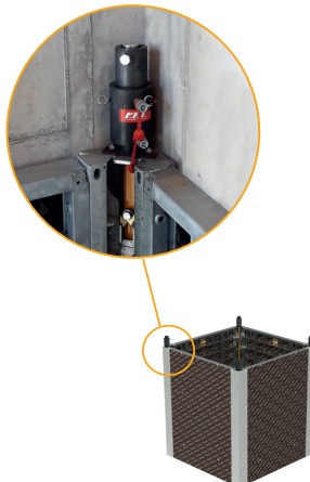
Hydraulisk operasjon
